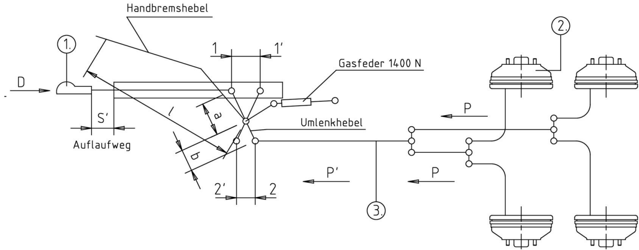
Schema der Auflaufbremsanlage
